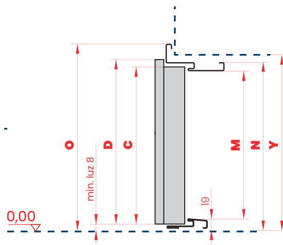
PRZEKRÓJ PIONOWY
