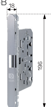
ZAMEK CHROM MAT Z SZARĄ NAKŁADKĄ Z LOGO I SREBRNĄ BLACHĄ ZACZEPOWĄ
