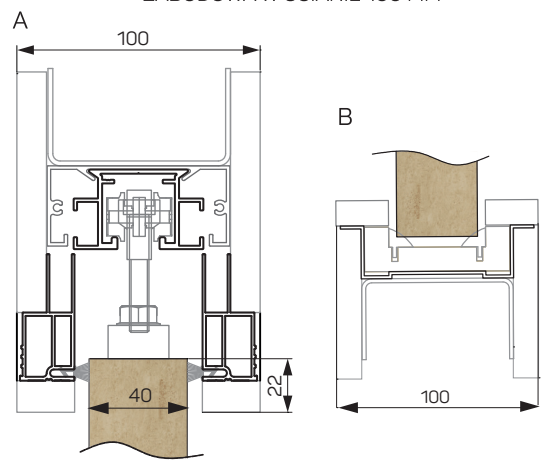
ZABUDOWA W ŚCIANIE 100 MM
