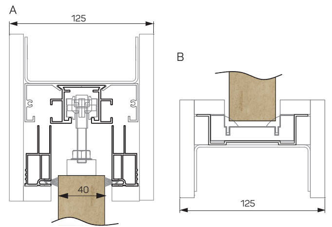
ZABUDOWA W ŚCIANIE 125 MM
