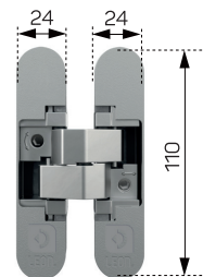
SZARY ZAWIAS Z SZARĄ NAKŁADKĄ
