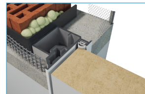
DRZWI ZEWNĘTRZNE - ZABUDOWA MUR EXTERNAL DOORS - BRICK
