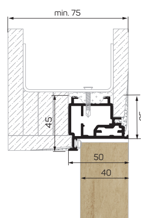
ZABUDOWA G-K / DRYWALL
