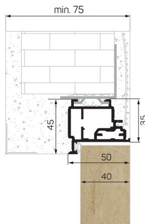
ZABUDOWA MUR / BRICK WALL
