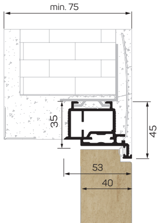
ZABUDOWA MUR / BRICK WALL
