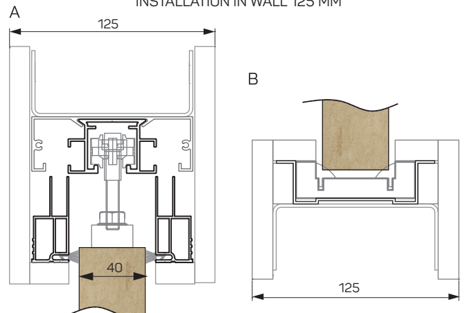
ZABUDOWA W ŚCIANIE 125 MM / INSTALLATION IN WALL 125 MM
