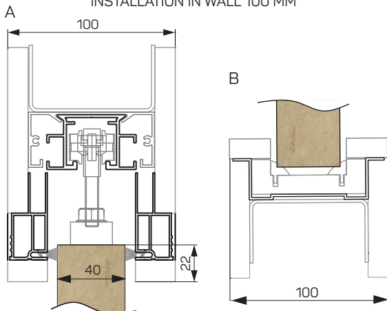
ZABUDOWA W ŚCIANIE 100 MM / INSTALLATION IN WALL 100 MM
