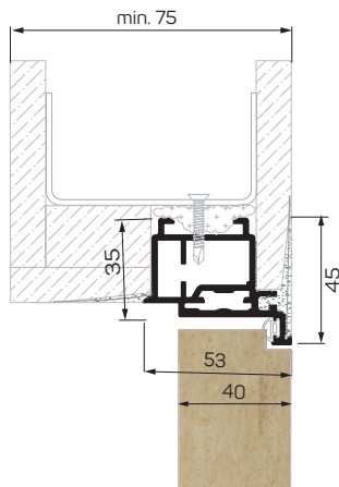
ZABUDOWA G-K / DRYWALL
