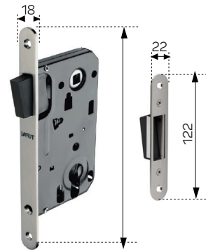
ZAMEK NIKIEL LOCK NICKEL
