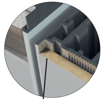
SKRZYDŁO BEZ RANTU
