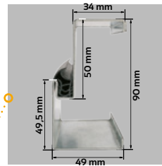
PRZEKRÓJ OŚCIEŻNICY SYMETRYCZNEJ Z USZCZELKĄ
