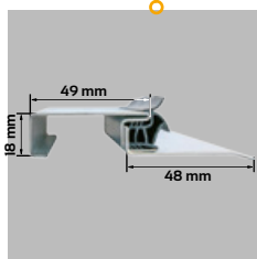
PRÓG ZE STALI NIERDZEWNEJ Z USZCZELKĄ
