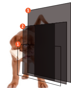
Antisol grafit + aplikacja mleczna 1 - szyba bezbarwna 2 - antisol grafit + folia mleczna 3 - szyba bezbarwna
